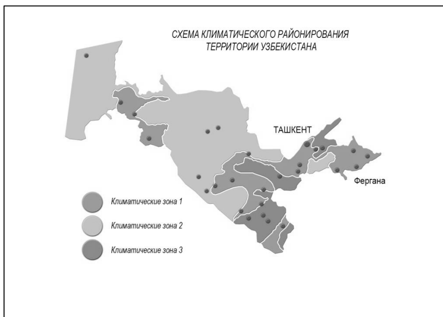
Рис. 2. Схема климатического районирования территории Узбекистана
